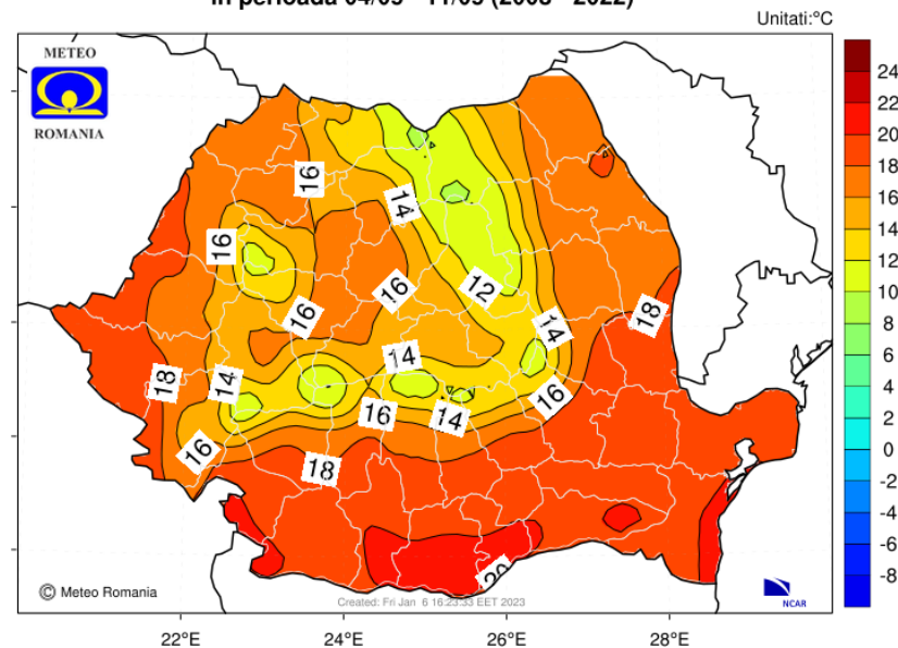
Media multianuala a temperaturii aerului la 2 m in perioada 04/09 - 11/09 (2003 - 2022)
