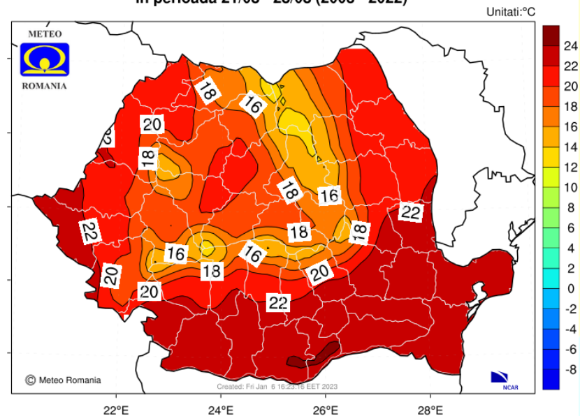
Media multianuala a temperaturii aerului la 2 m in perioada 21/08 - 28/08 (2003 - 2022)
