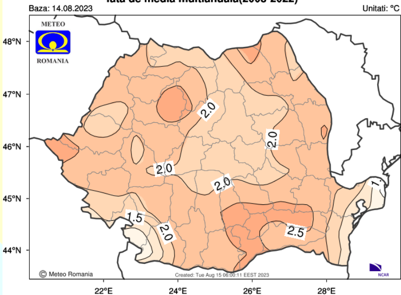
Abaterea temperaturii medii a aerului in perioada 21/08/2023 - 28/08/2023 fata de media multianuala(2003-2022)
